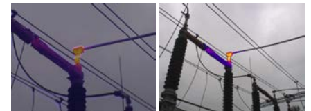
Überblendung Wärme-/Sichtbild Farbalarm
