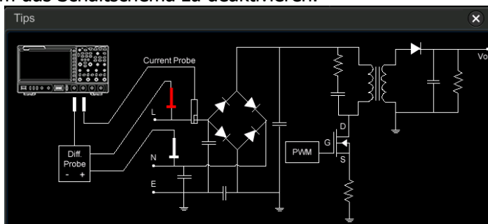
Bild 8-1 Typisches Schaltschema Leistungsqualitätsanalyse (Connection Diagram of Power Quality Analysis)
